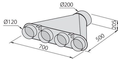
可连接4条管的歧管 2525 000
